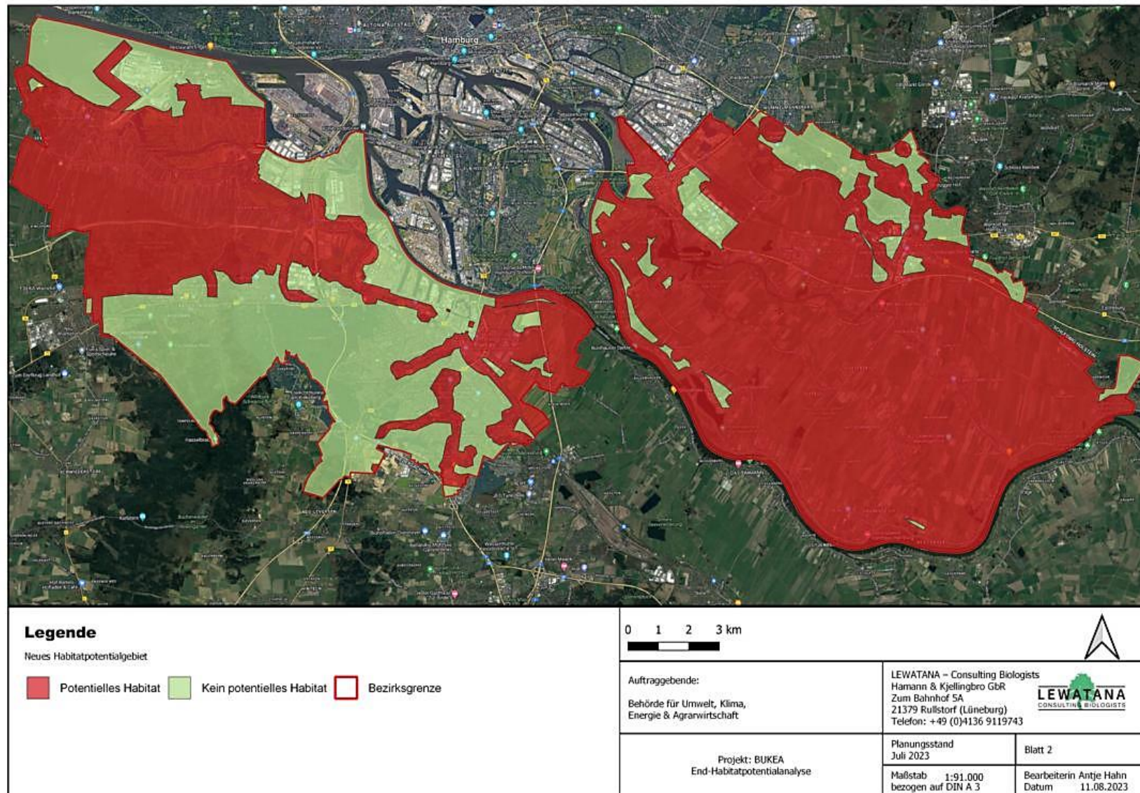
Abbildung 6: Endgültige Habitatpotentialanalyse für Nutria in den Bezirken Harburg und Bergedorf.
