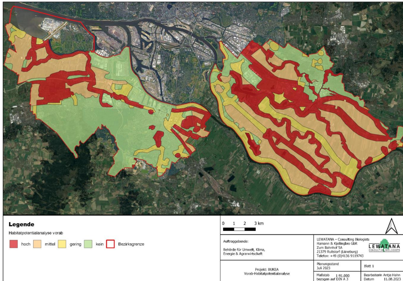
Abbildung 5: Vorab-Habitatpotentialanalyse mit Einstufung des Habitatpotentials für Nutria.
