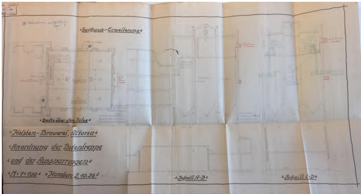
Abb. 35: Schnitte Sudhaus-Erweiterung 1926
