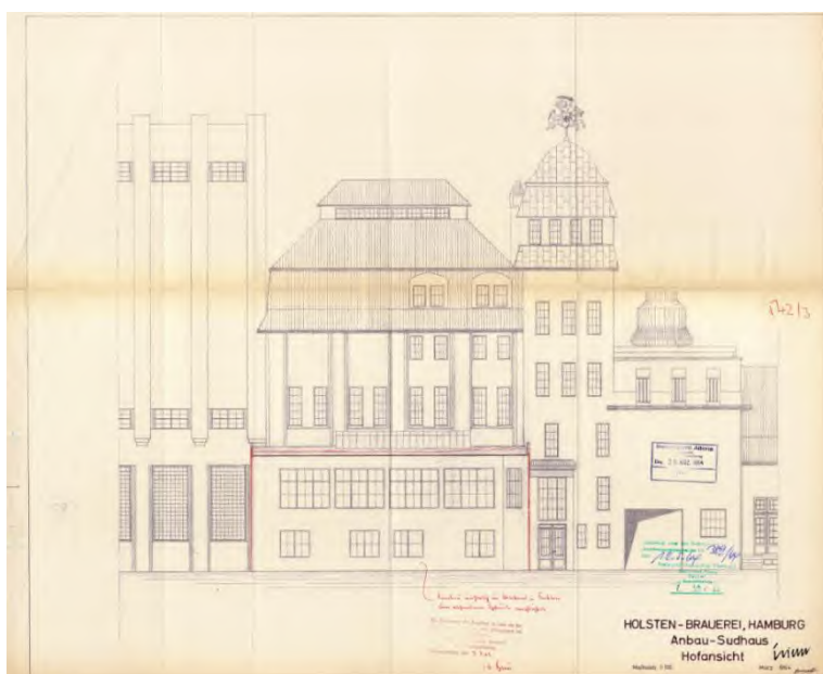
Abb. 27: Anbau Sudhaus 1964 - Hofansicht
