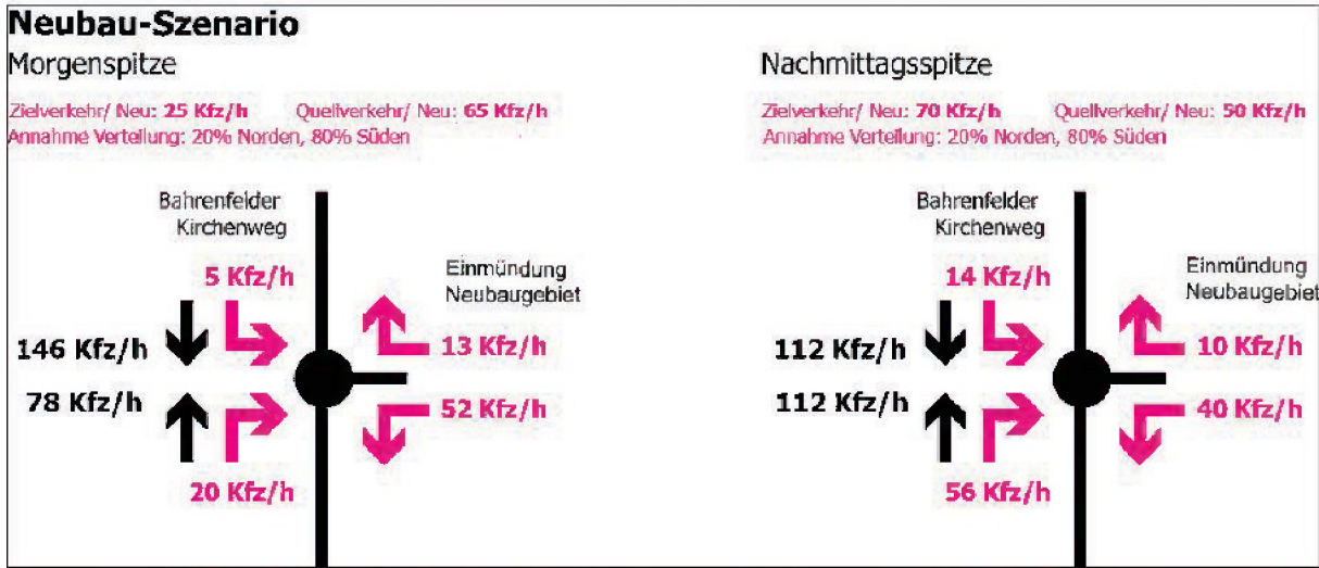
Abbildung 11: Knotenströme für Neubau-Szenario am Knotenpunkt Bahrenfelder Kirchenweg/ Anbindung Euler-Hermes-Areal
