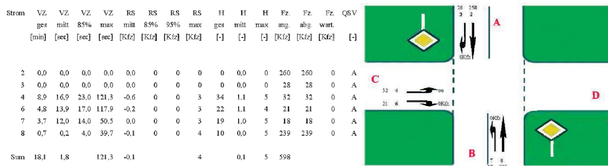
Abbildung 22: Leistungsfähigkeitsnachweis Nachmittagspitze Knotenpunkt Hohenzollernring/ Anbindung Henkel-Areal Nord
