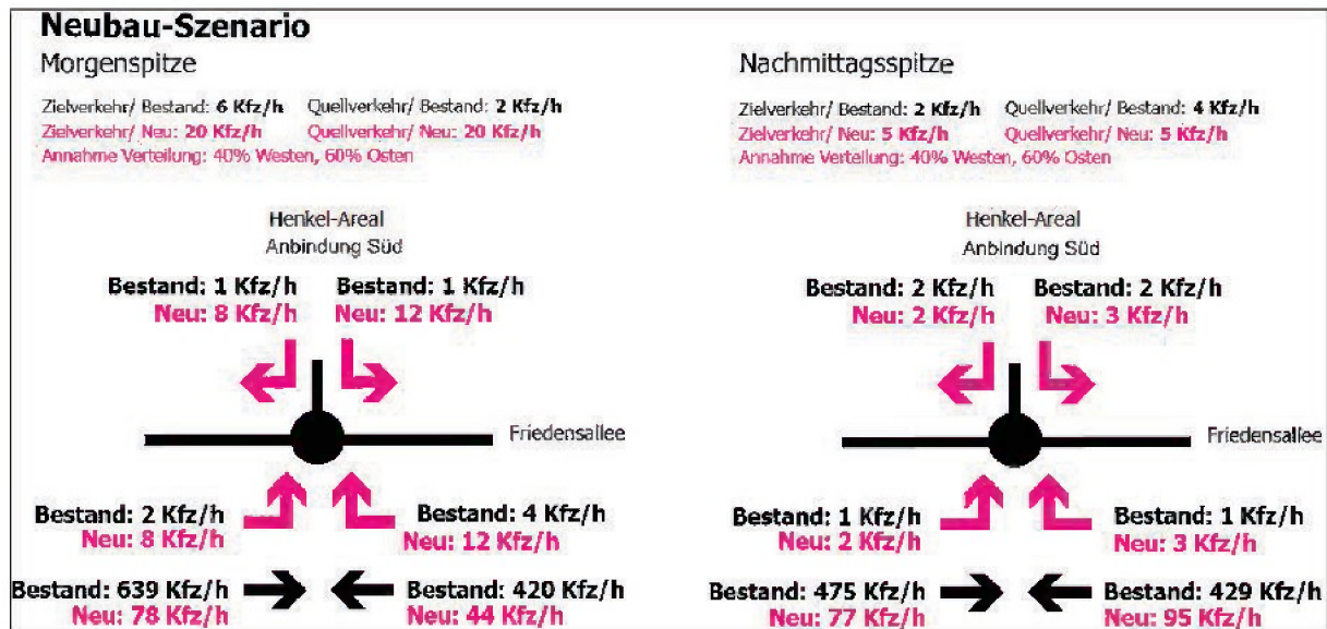
Abbildung 17: Knotenströme für Neubau-Szenario am Knotenpunkt Friedensallee/ Anbindung Henkel-Areal Süd
