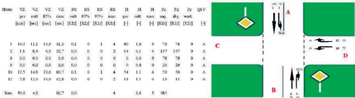
Abbildung 12: Leistungsfähigkeitsnachweis Morgenspitze Knotenpunkt Bahrenfelder Kirchenweg/ Anbindung Euler-Hermes-Areal
