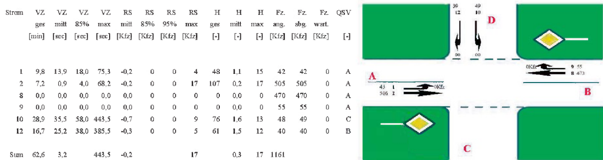
Abbildung 16: Leistungsfähigkeitsnachweis Nachmittagsspitze Knotenpunkt Friedensallee/ Anbindung Kolbenschmidt-Areal
