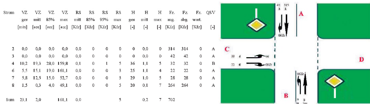
Abbildung 21: Leistungsfähigkeitsnachweis Morgenspitze Knotenpunkt Hohenzollernring/ Anbindung Henkel-Areal Nord
