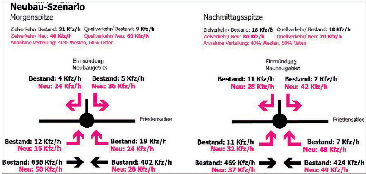
Abbildung 14: Knotenströme für Neubau-Szenario am Knotenpunkt Friedensallee/ Anbindung Kolbenschmidt-Areal
