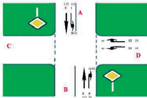
Abbildung 13: Leistungsfähigkeitsnachweis Nachmittagsspitze Knotenpunkt Bahrenfelder Kirchenweg/Anbindung Euler-Hermes-Areal
