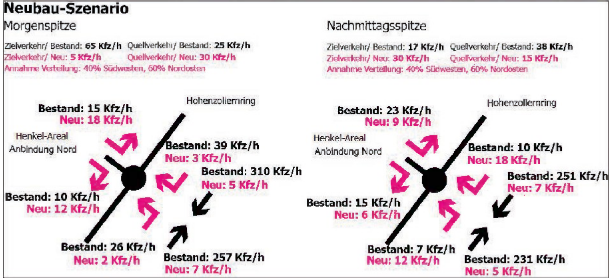
Abbildung 20: Knotenströme für Neubau-Szenario am Knotenpunkt Hohenzollernring/ Anbindung Henkel-Areal Nord
