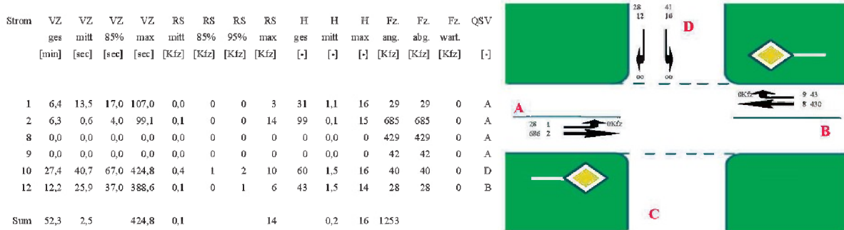
Abbildung 15: Leistungsfähigkeitsnachweis Morgenspitze Knotenpunkt Friedensallee/ Anbindung Kolbenschmidt-Areal
