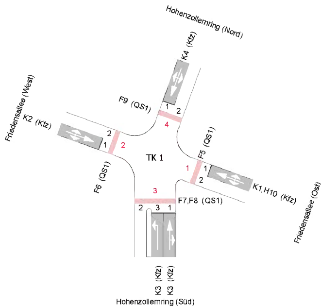
Abbildung 24: Übersicht Knotenpunkt Hohenzollernring/ Friedensallee
