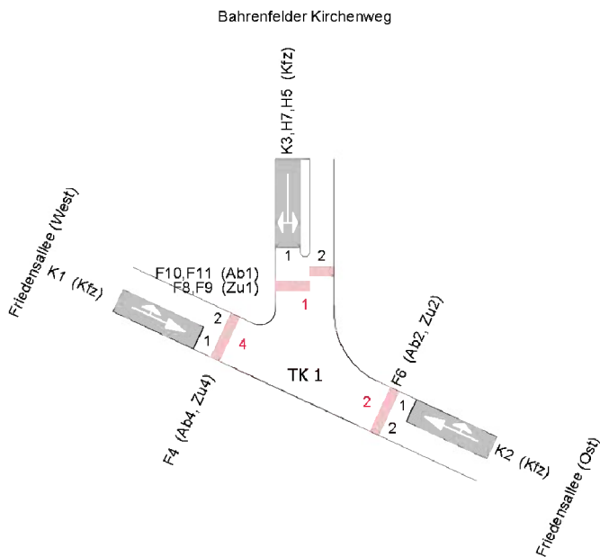
Abbildung 23: Übersicht Knotenpunkt Friedensallee/ Bahrenfelder Kirchenweg
