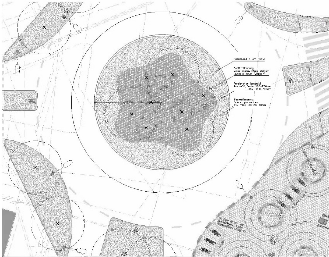
Detailplan Kreisverkehr mit Sprunginseln M 1:100
