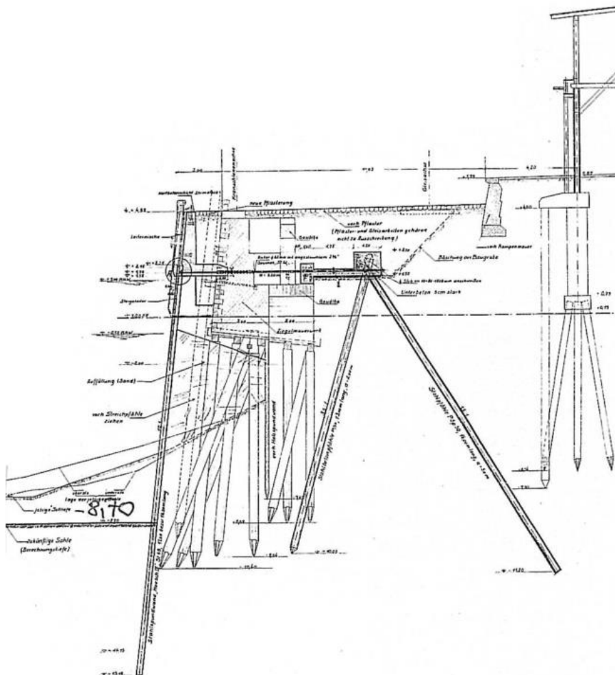
Abb. 59: Kaimauerverstärkung am Asiakai, 1954 bis 1964, Ausschnitt (Quelle: Hamburg Port Authority AÖR (HPA))
