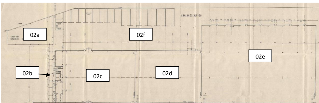
Abb. 124: Hallenabschnitte 02a bis 02f, Grundriss, Stand 1984, Ausschnitt (Quelle: Hamburger Hafen und Logistik AG (HHLA))
