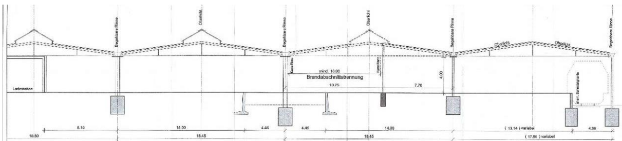
Abb. 123: Hallenabschnitt 02g, Querschnitt Nord-Süd-Richtung, Blickrichtung Osten, Stand 2005, Ausschnitt (Quelle: Hamburger Hafen und Logistik AG (HHLA))
