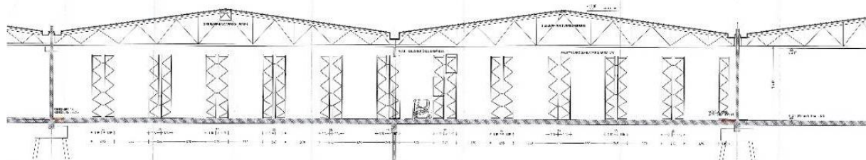
Abb. 120: Hallenabschnitte 01c (links) und 01b (rechts), ganz links Hallenabschnitt 01d, ganz rechts Hallenabschnitt 01a, Schnitte, Stand 2013, Ausschnitt (Quelle: Hamburger Hafen und Logistik AG (HHLA))
