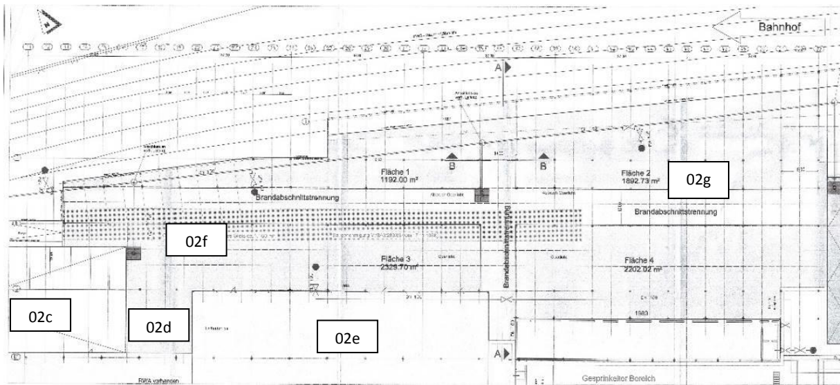
Abb. 122: Hallenabschnitte 02d bis 02g, Grundriss, Stand 2005, Ausschnitt. Die Hallenabschnitte 02a und 02b liegen im Westen und sind hier nicht dargestellt. (Quelle: Hamburger Hafen und Logistik AG (HHLA))
