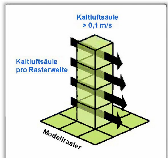
Abb. 8: Prinzipskizze Kaltluftvolumenstrom
